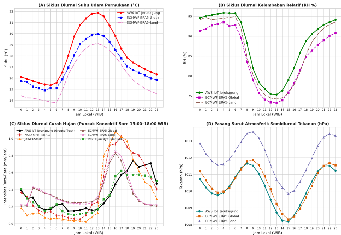
Gambar 5: Siklus Diurnal Rata-Rata 24-Jam: (A) Suhu Udara Permukaan, (B) Kelembaban Relatif, (C) Presipitasi (6 Sumber Data Jam-Jaman), dan (D) Pasang Surut Semidiurnal Tekanan Udara di Stasiun Jerukagung Kebumen.
