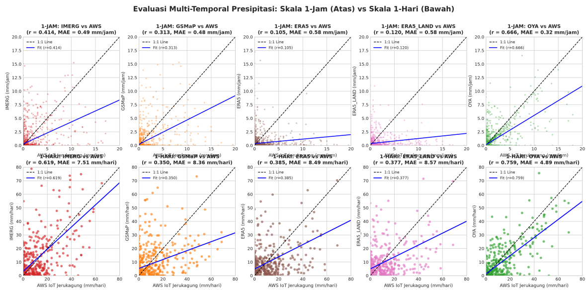
Gambar 3: Diagram Pencar Multi-Skala Konsisten 2 \times 5 : Resolusi 1-Jam (Atas) vs Resolusi 1-Hari (Bawah) Lengkap dengan Garis 1:1 dan Regresi Linier.
