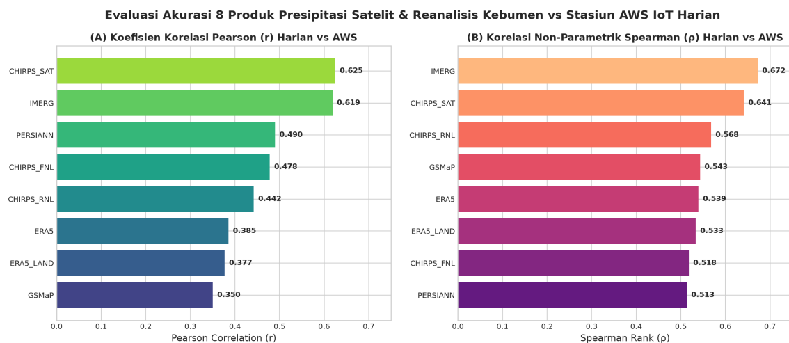
Gambar 1: Peringkat Koefisien Korelasi Linier Pearson ( r ) dan Rank Spearman ( \rho ) Seluruh Produk Satelit dan Reanalisis Harian terhadap AWS IoT Jerukagung.
