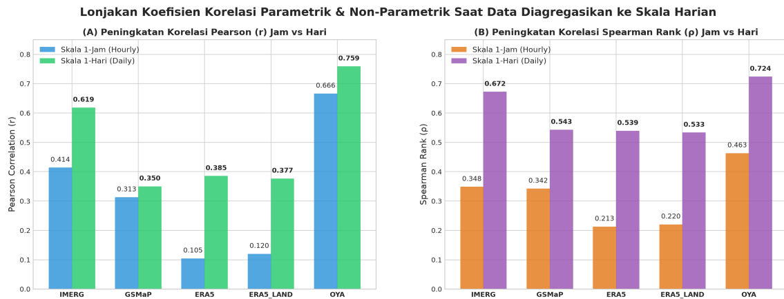
Gambar 4: Lonjakan Koefisien Korelasi Parametrik Pearson ( r ) dan Non-Parametrik Spearman ( \rho ) Saat Data Diagregasikan ke Skala Harian.
