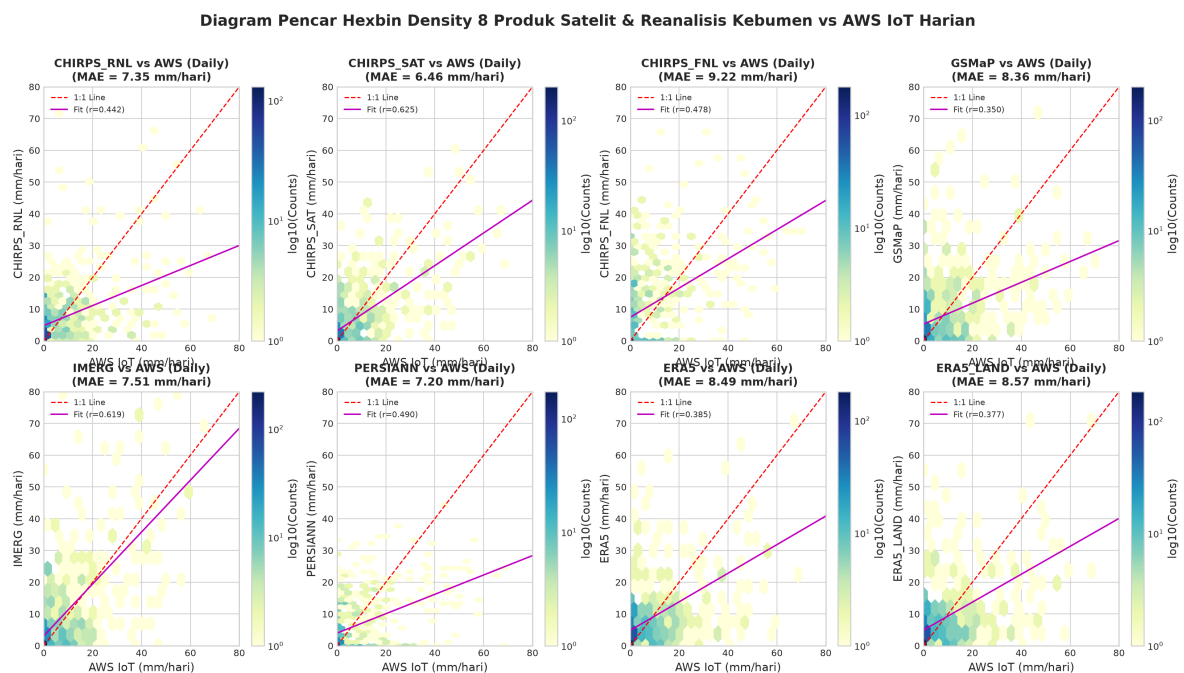
Gambar 2: Diagram Pencar Kepadatan Logaritmik ( Hexbin Density Scatter ) 8 Produk Presipitasi Satelit & Reanalisis Kebumen vs AWS IoT Harian.
