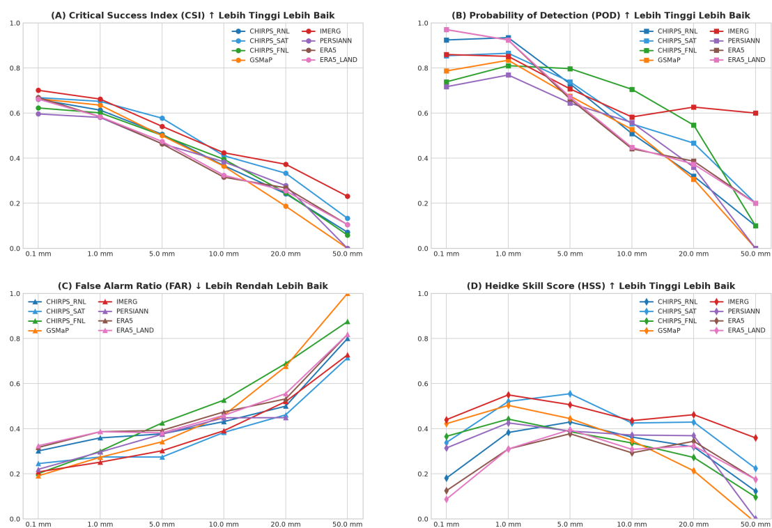
Gambar 6: Kurva Metrik Kontingensi Deteksi Hujan Harian: (A) CSI, (B) POD, (C) FAR, dan (D) HSS pada Berbagai Ambang Batas Intensitas (0,1 – 50 mm/hari) terhadap AWS IoT.
