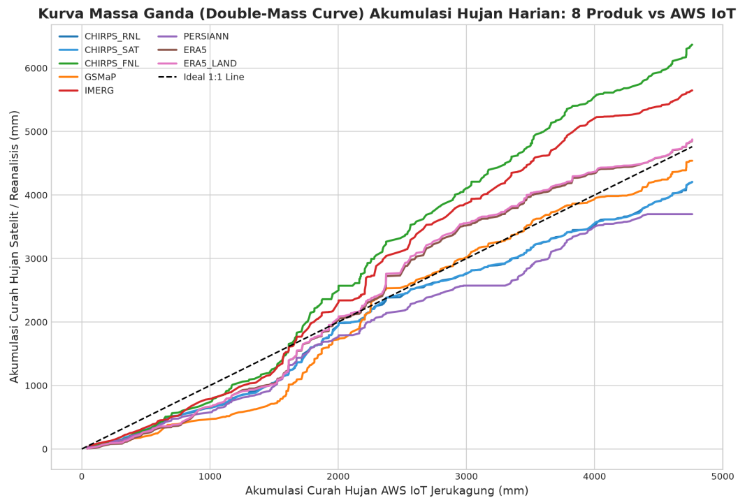
Gambar 7: Kurva Massa Ganda ( Double-Mass Curve ) Akumulasi Curah Hujan Harian 8 Produk Satelit terhadap Stasiun AWS IoT Jerukagung.
